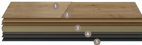
Aufbau HARO TRITTY 250
