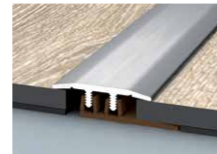
Übergangprofil Profi-Design Zweiteiliges Aluminiumprofil zur Überdeckung von Dehnungsfugen
