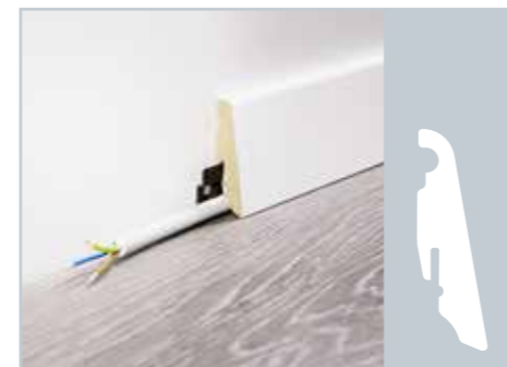
Fußleiste 19/58 MDF-Träger 19 × 58 × 2400 mm VE = 4 Stück
