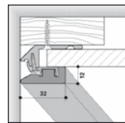
Abschlussleiste
