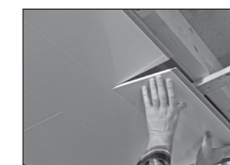
Klick-Paneele einschwenken
