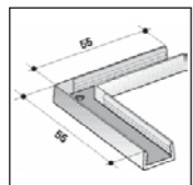
Eckverbinder HDF-Leiste
